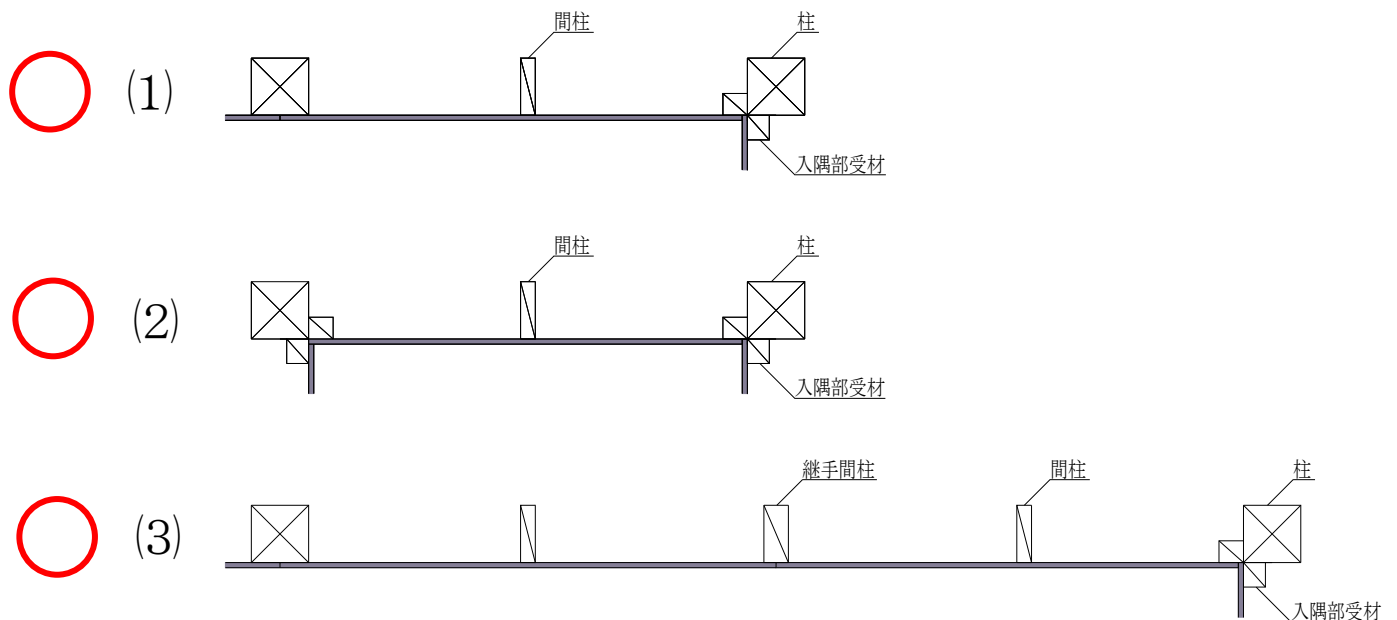
図 9 入隅部の納まり図①
