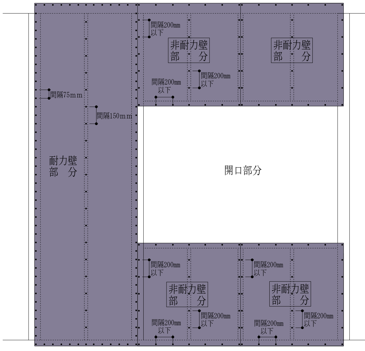
図 17 耐力壁・非耐力壁 納まり図
